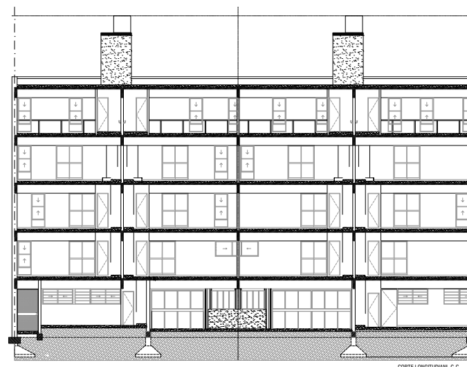
Corte longitudinal C-C
