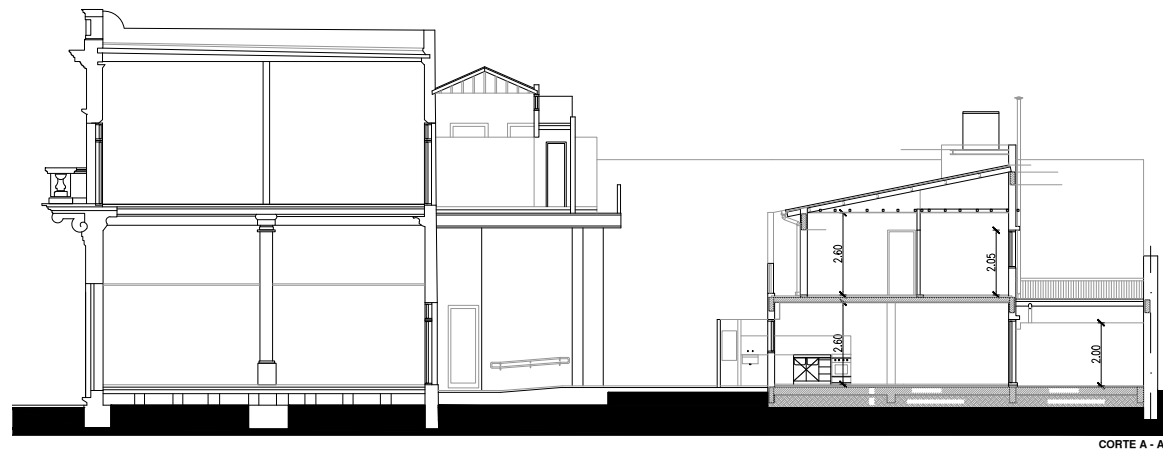
Cortes
