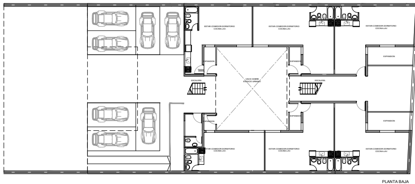
Planta baja
