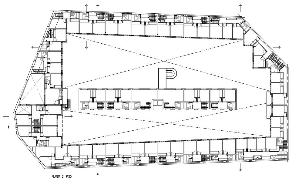
Planta 2do piso
