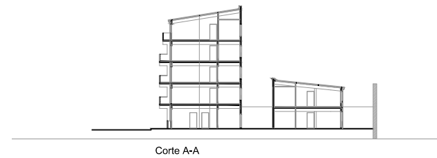
Corte A-A
