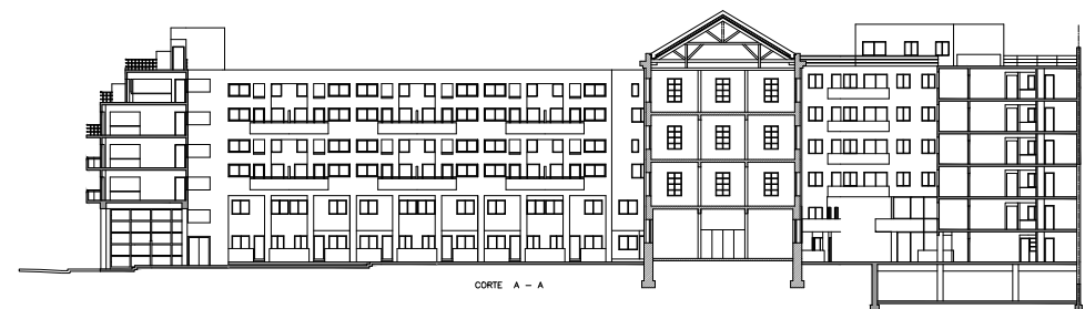
Corte A-A
