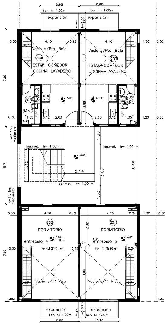
Planta 2do piso
