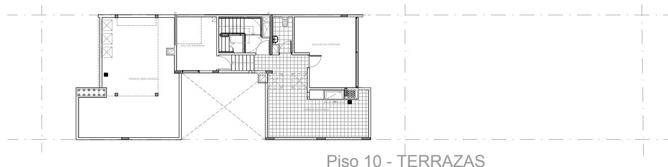
Planta 10mo piso - Terrazas
