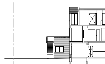
Corte transversal
