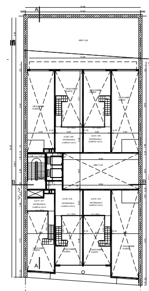
Planta entrespiso 2do y 3er piso
