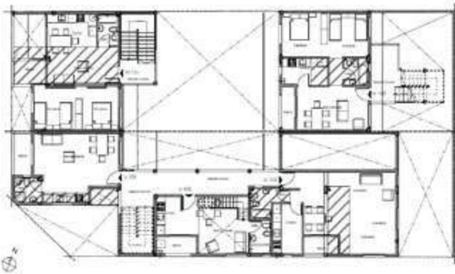
Planta 1er piso
