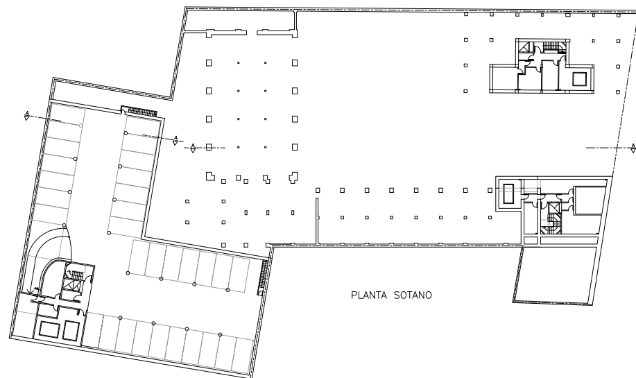
Planta sótano
