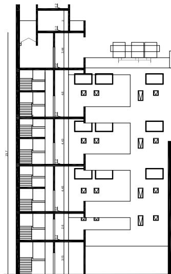
Corte longitudinal
