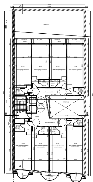
Planta 1er piso
