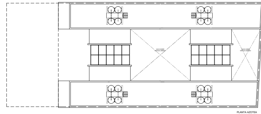
Planta azotea
