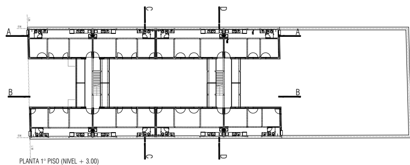
Planta baja (Nivel) Planta 1er piso (Nivel + 3.00)
