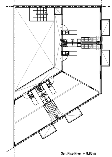
3er piso. Nivel + 8,80 m.
