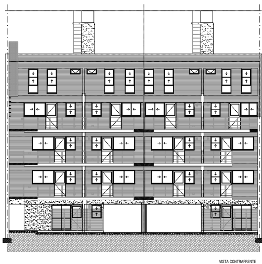
Vista contrafrente
