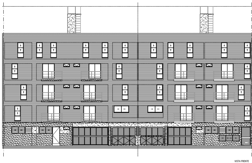
Vista frente
