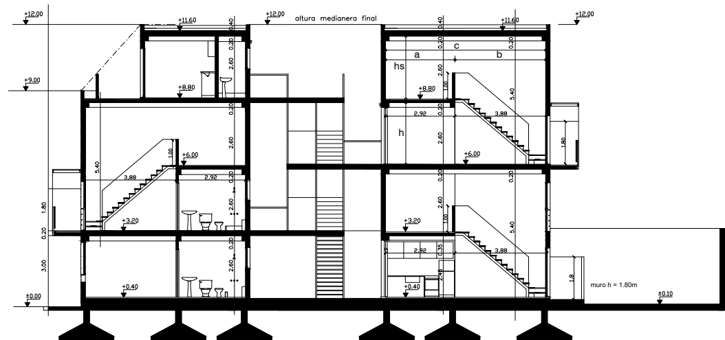
Corte
