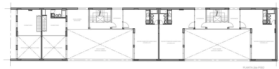
Planta 2do piso
