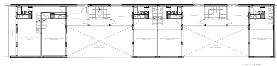
Planta 3er piso
