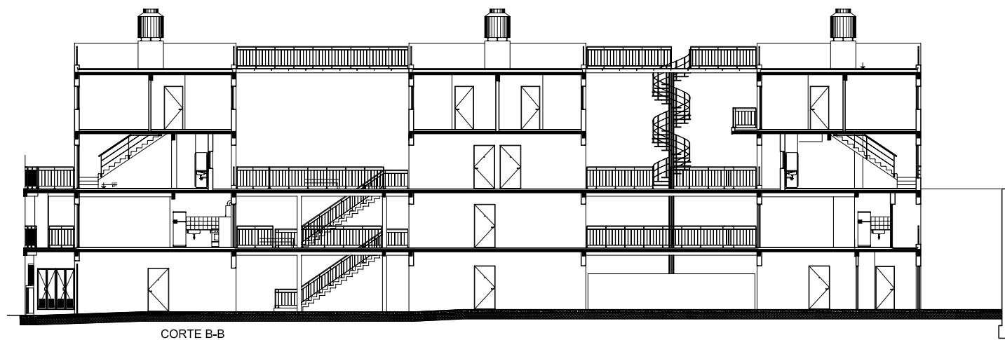
Corte
