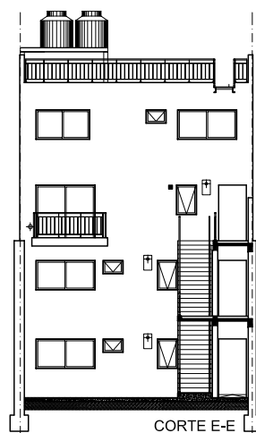
Corte
