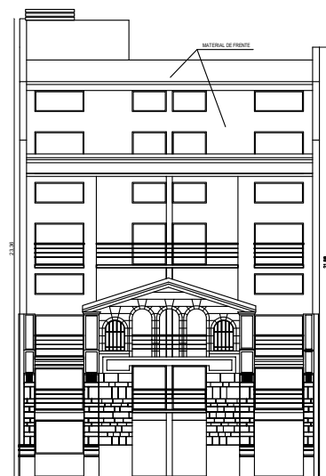
Fachada
