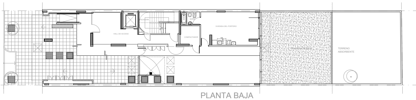
Planta baja
