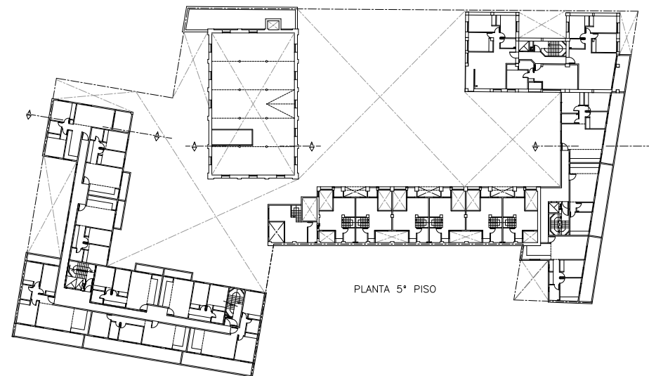
Planta 5to piso
