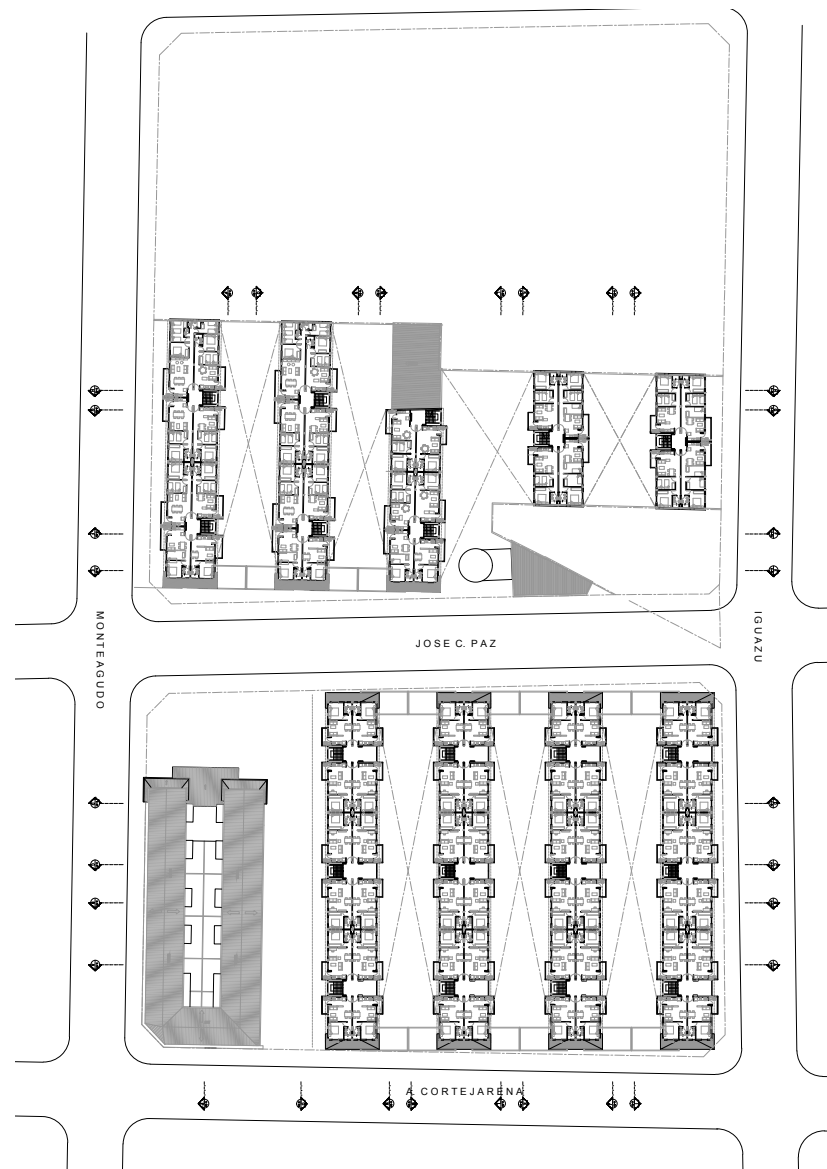
Planta 3er piso
