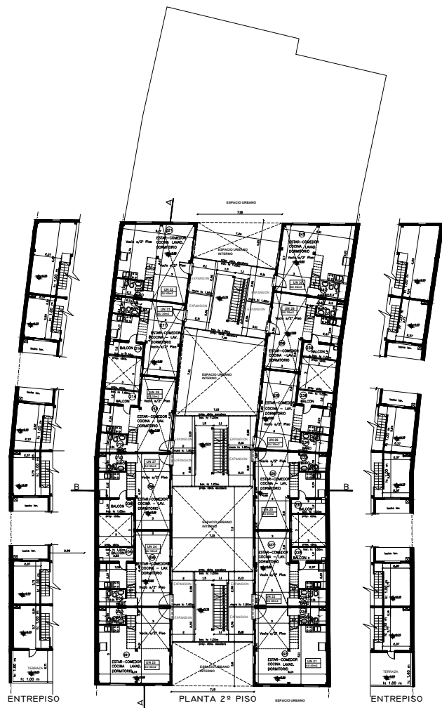
Plantas 2do piso y entrepisos
