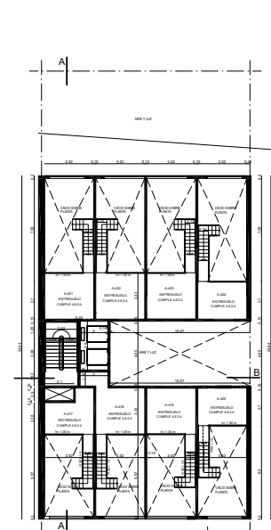
Planta entrespiso 4to piso
