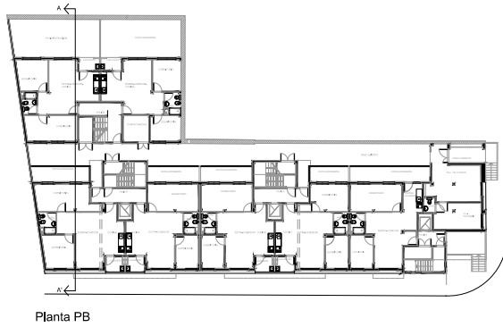
Planta baja
