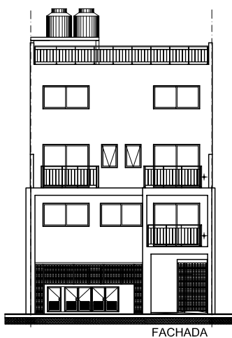
Fachada
