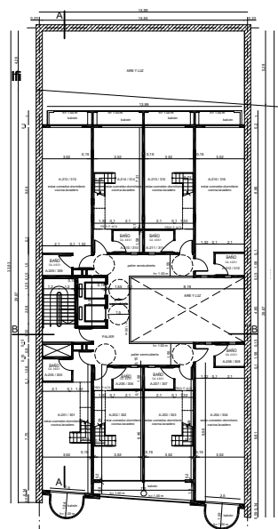
Planta 3er piso
