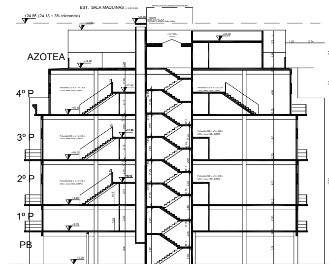
Corte transversal
