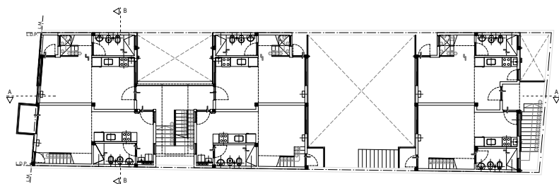
Plantas
