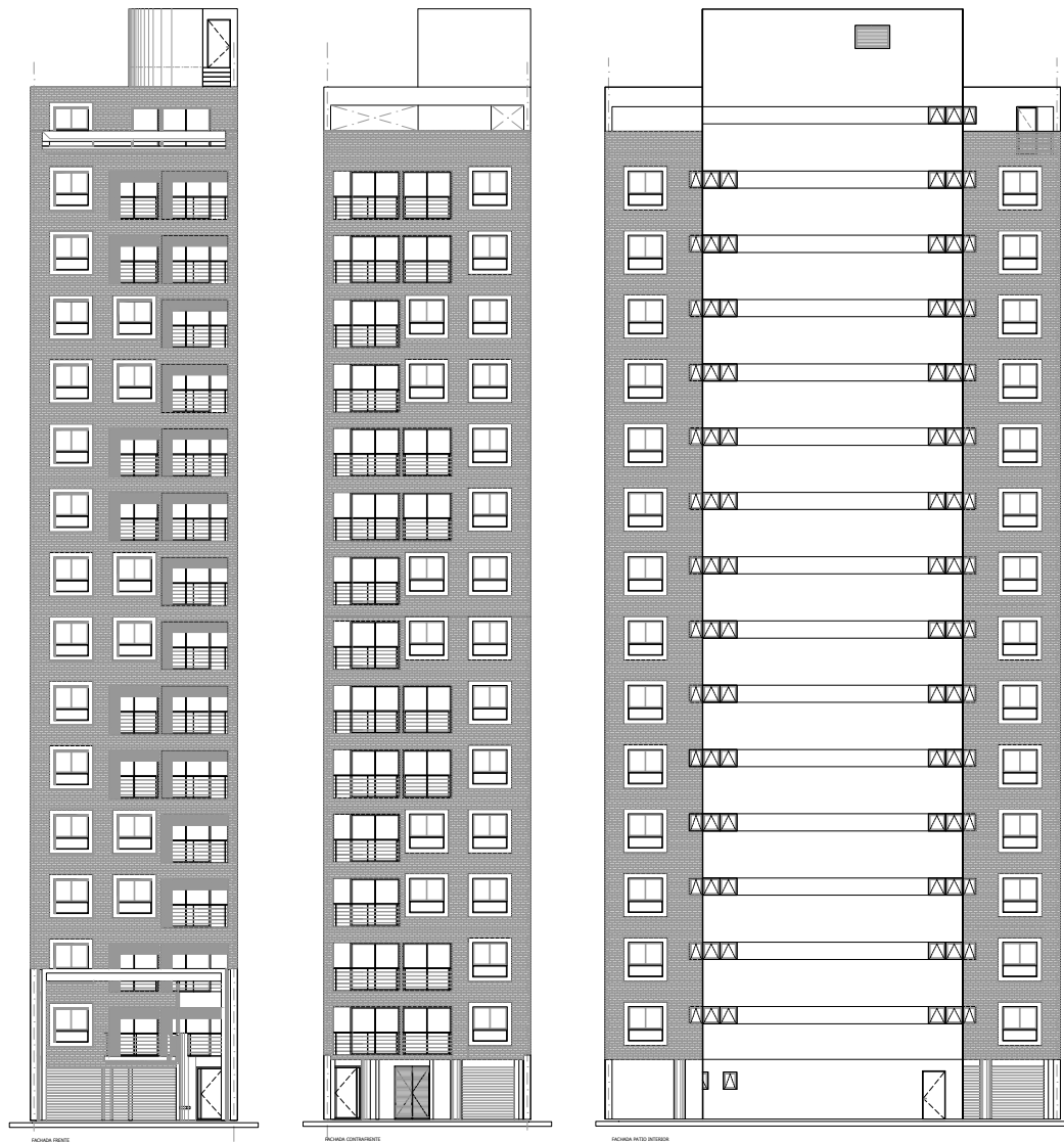
Vistas frente y contrafrente
