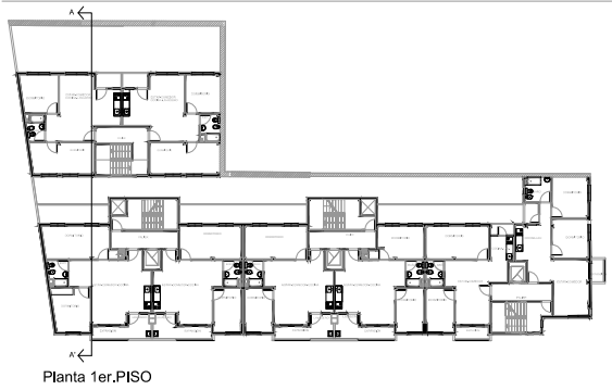
Planta 1er piso
