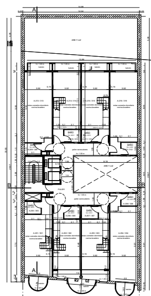
Planta 2do piso
