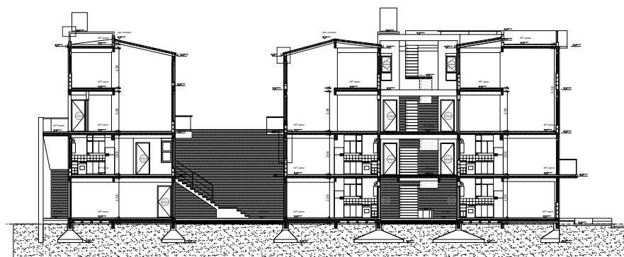
Corte
