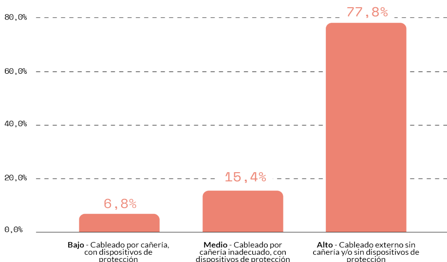
Gráfico 1: Exposición a riesgo eléctrico, según tipo de instalación domiciliaria
